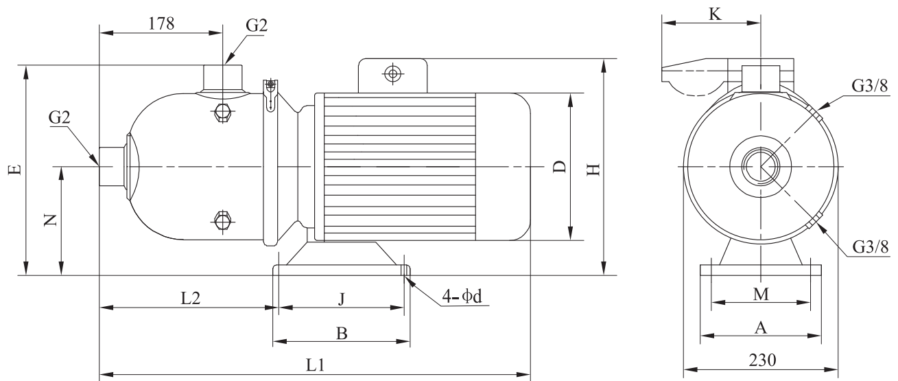
Габаритно-присоединительные размеры и масса
