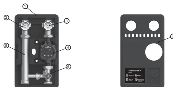
Рис. 2 Насосная группа с 3-ходовым смесительным клапаном
