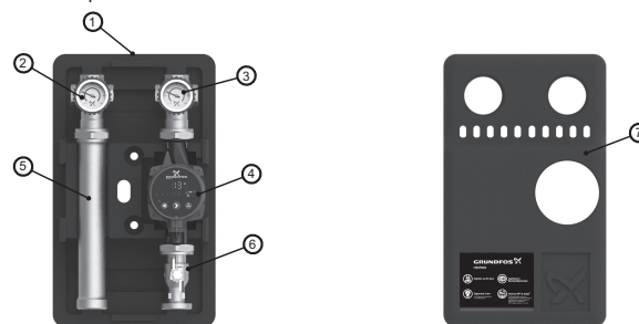
Рис. 1 Насосная группа с прямым контуром
